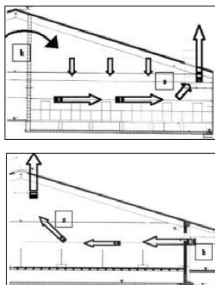
Figure 1 : points de prélèvement en fonction du circuit d'air dans le bâtiment (Costa, 2007)
