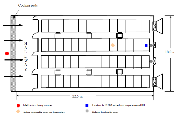
Figure 2 : Points de prélèvement d'air (Jerez et al. 2005)
