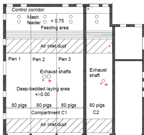
Figure 2 : Points de prélèvement d'air (+) en salle d'engraissement (Haeussermann, 2007)
