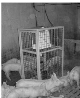
Figure 4 : Cage dans laquelle se trouve l'appareil de mesure (Van Ransbeeck, 2012)
